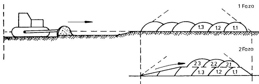
Rys. 1. Schemat zdjęcia ziemi urodzajnej za pomocą spycharki z przesunięciem jej na zwałę (wg S. Datka, S. Lenczewski: Drogowe roboty ziemne, WKŁ 1979)
