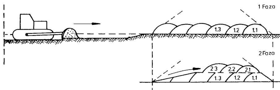
Rys. 1. Schemat zdjęcia ziemi urodzajnej za pomocą spycharki z przesunięciem jej na zwałę (wg S. Datka, S. Lenczewski: Drogowe roboty ziemne, WKŁ 1979)
