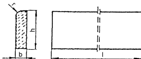
Rysunek 1. Kształt obrzeża chodnikowego betonowego
