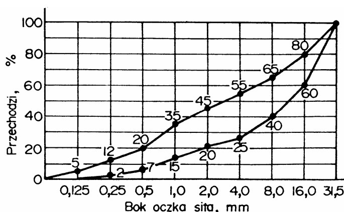
Rysunek 1. Graniczne krzywe uziarnienia mieszanki betonowej od 0 do 31,5 mm.
