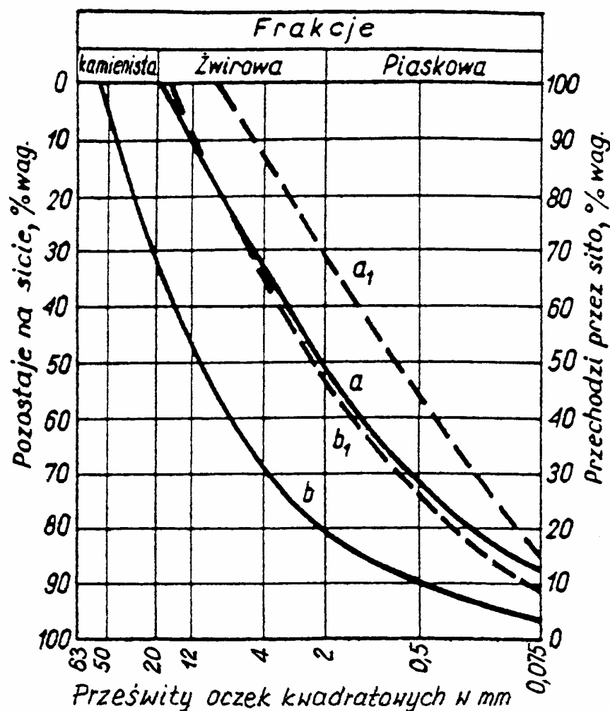
Rysunek 5.1. Obszar uziarnienia optymalnych mieszanek żwirowych
